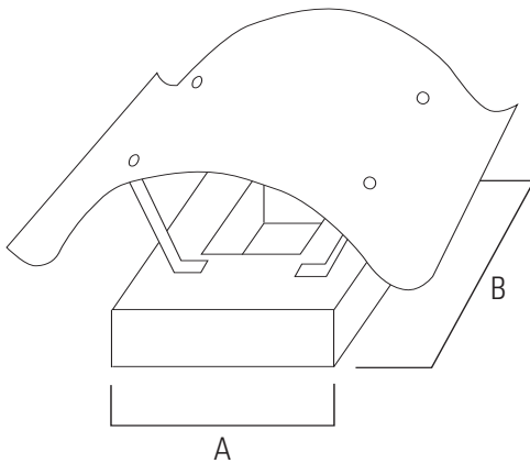
Grömo Kaminhaube, Napoleonform mit Verstärkungssicken, 1mm stark, incl. Kaminfüße und Befestigungsset.
